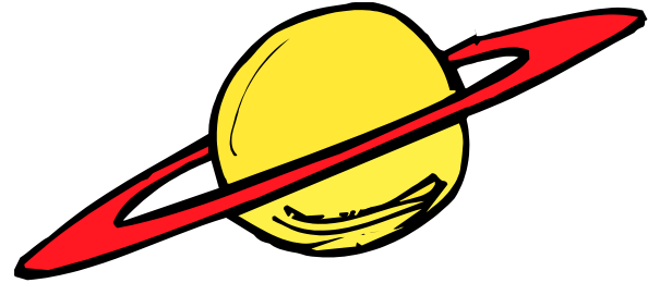
planet
