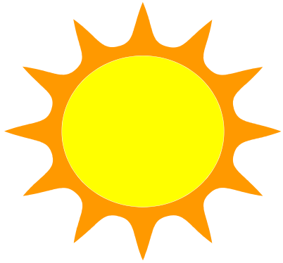
sun
