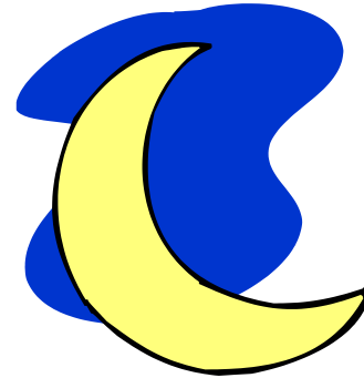
moon
